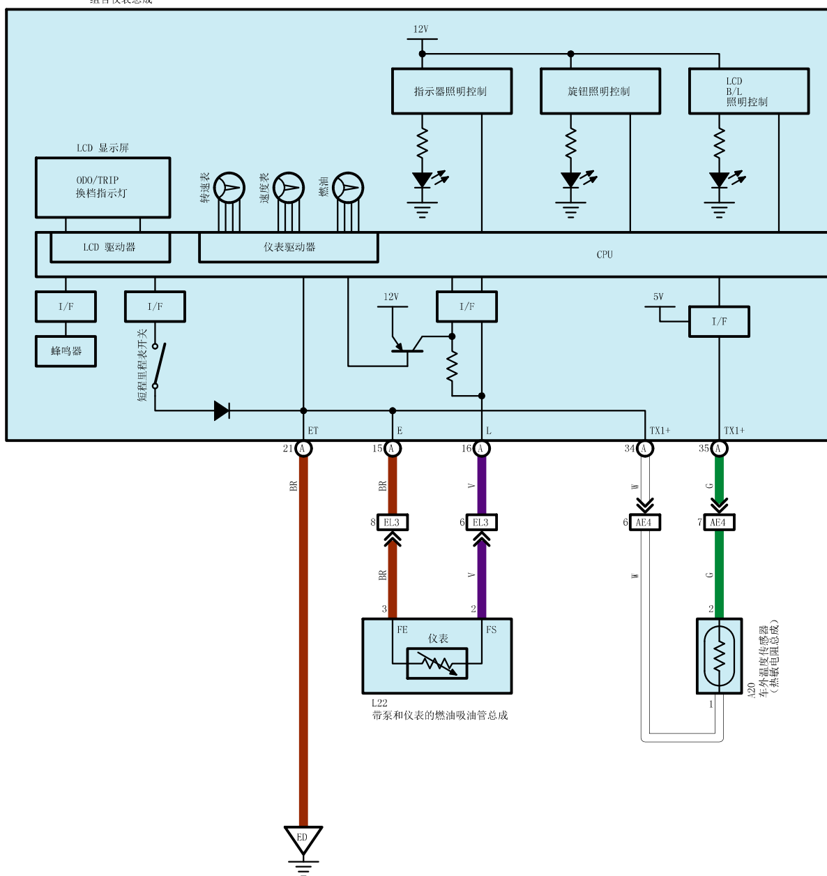
E55 (A), E59 (B) 组合仪表总成
